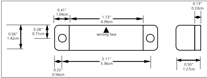
ACTUATOR
